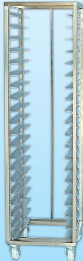
烤盤架車 Tray Holder 外徑 External Size 52x72x183cm 50x70x183cm
